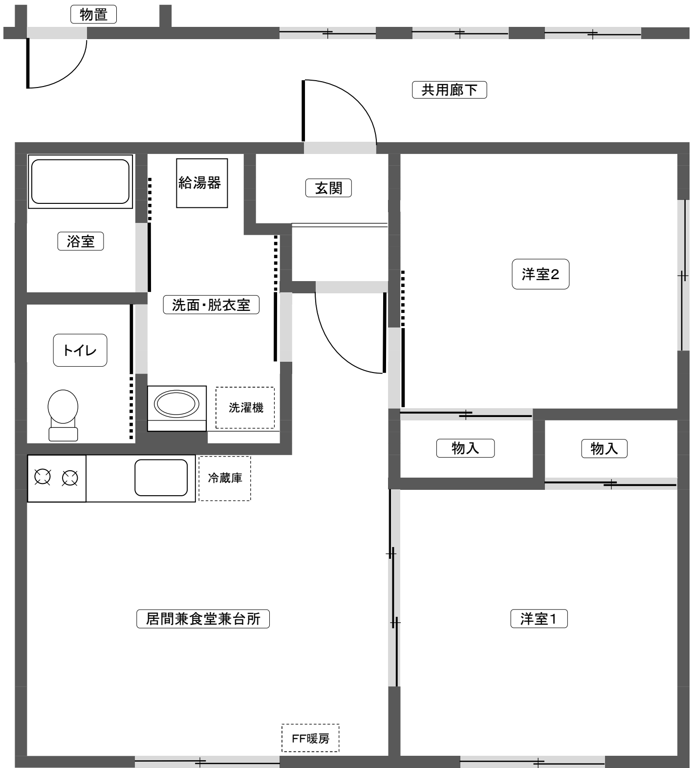
あけぼの団地1号・2号棟間取り図
